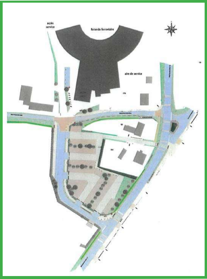
Plan d'aménagement du parking de la Rotonde
